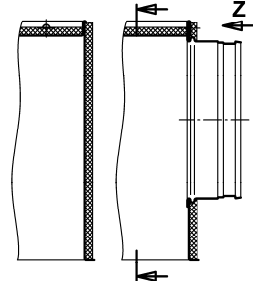
external (-Ia)
