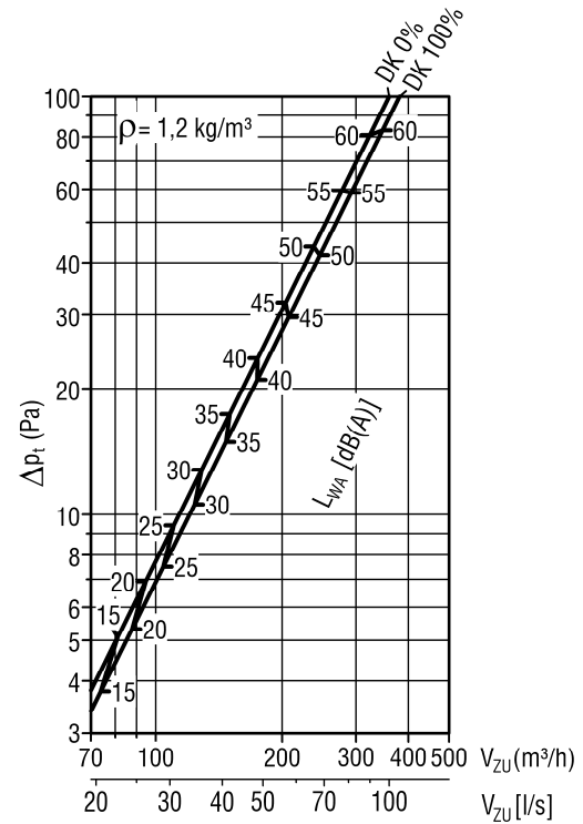
CDD-M-K/-E-...-Z-...
