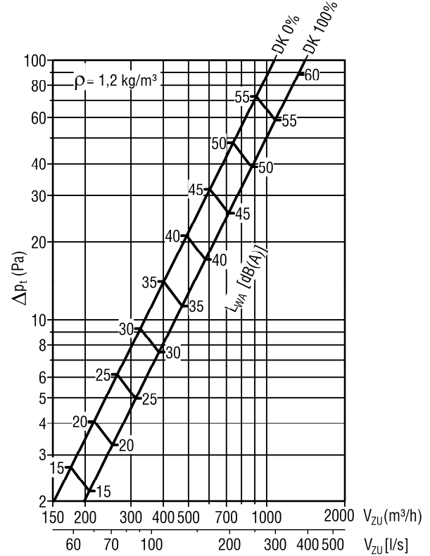
CDD-M-K/-E-...-Z-...
