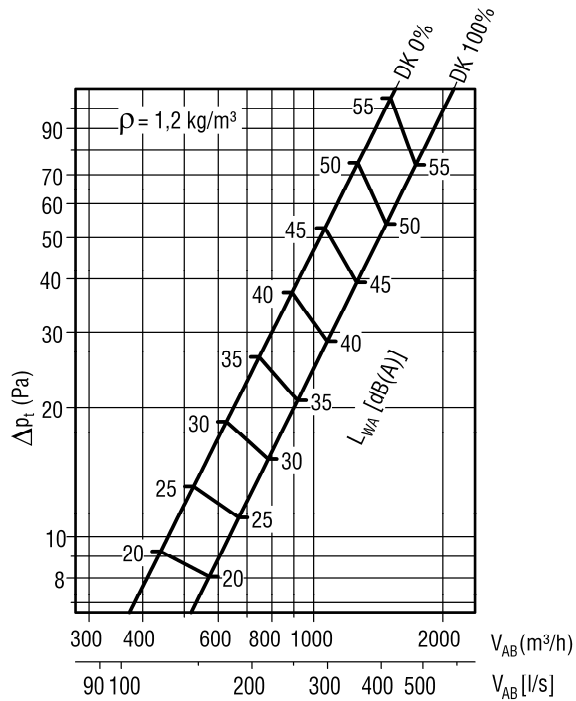
CDD-N-K/E-...-A-...
